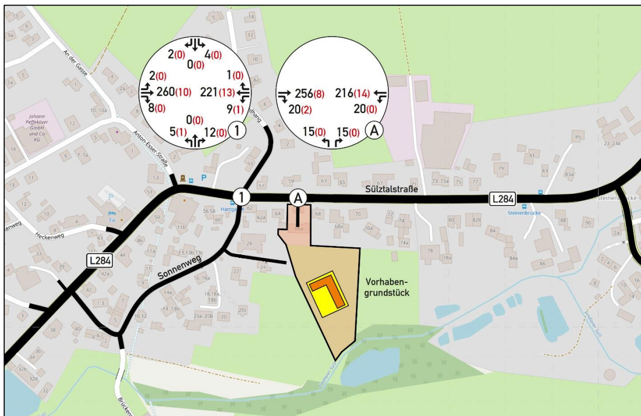
Abbildung 14: Knotenstrombelastungen in der Morgenspitzenstunde im Analysefall PLUS [Kfz/h (SV/h)] (Kartengrundlage: OpenStreetMap – Mitwirkende 2023 [1])
