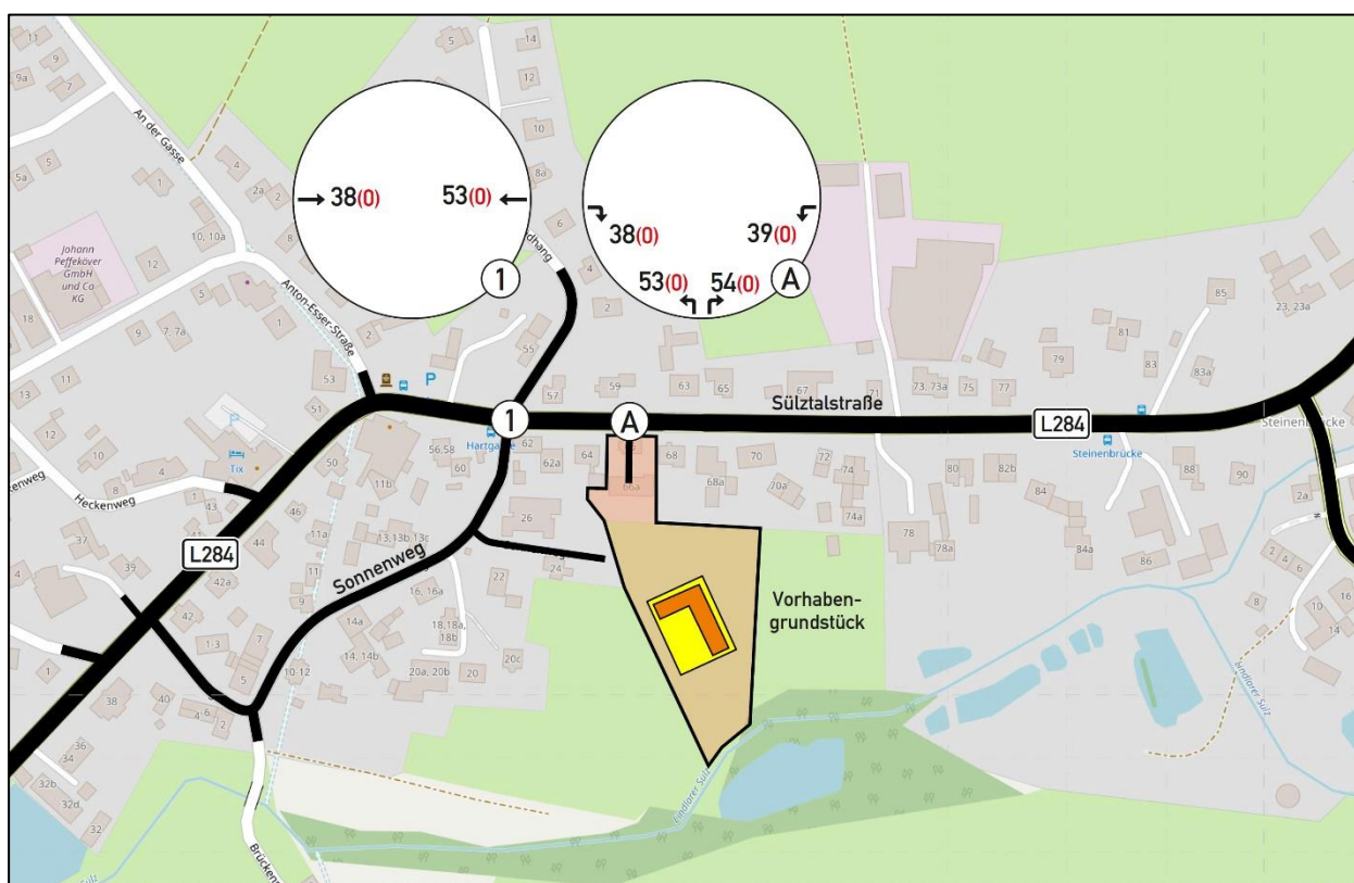
Abbildung 13: Verteilung der Neuverkehre in der Nachmittagspitzenstunde [Kfz/h] (Kartengrundlage: OpenStreetMap - Mitwirkende 2023 [1])
