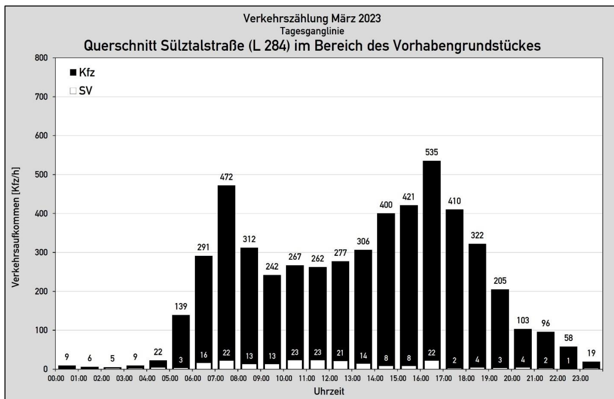
Abbildung 6: Tagesganglinie Querschnitt Sülztalstraße (L 284) [Kfz/h (SV/h)]
