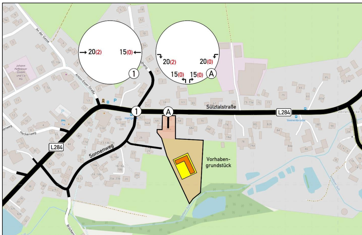
Abbildung 12: Verteilung der Neuverkehre in der Morgenspitzenstunde [Kfz/h] (Kartengrundlage: OpenStreetMap – Mitwirkende 2023 [1])
