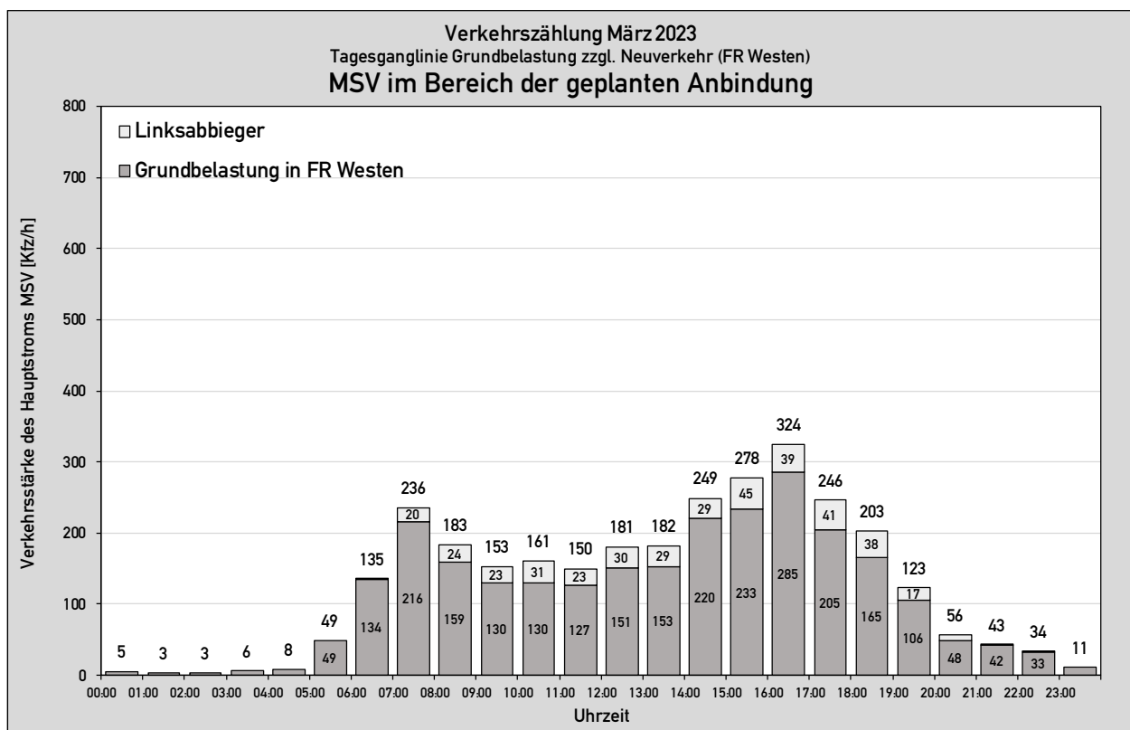
Abbildung 17: Tagesganglinie MSV für in Fahrtrichtung Norden fahrende Kfz in der Berliner Straße [Kfz/h]
