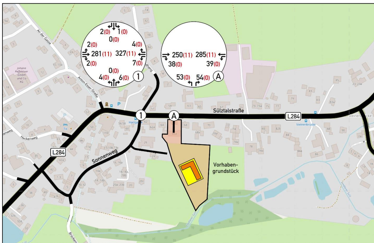
Abbildung 15: Knotenstrombelastungen in der Nachmittagspitzenstunde im Analysefall PLUS [Kfz/h (SV/h)] (Kartengrundlage: OpenStreetMap – Mitwirkende 2023 [1])
